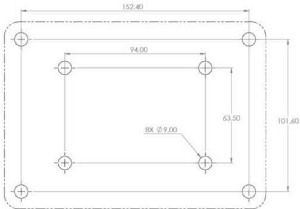
図 2-6 VR500 の底面ネジ穴レイアウト
