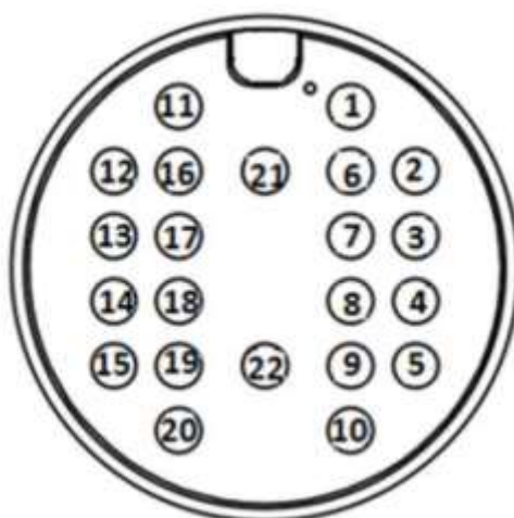
図 2-8 VR500 ピン配置
