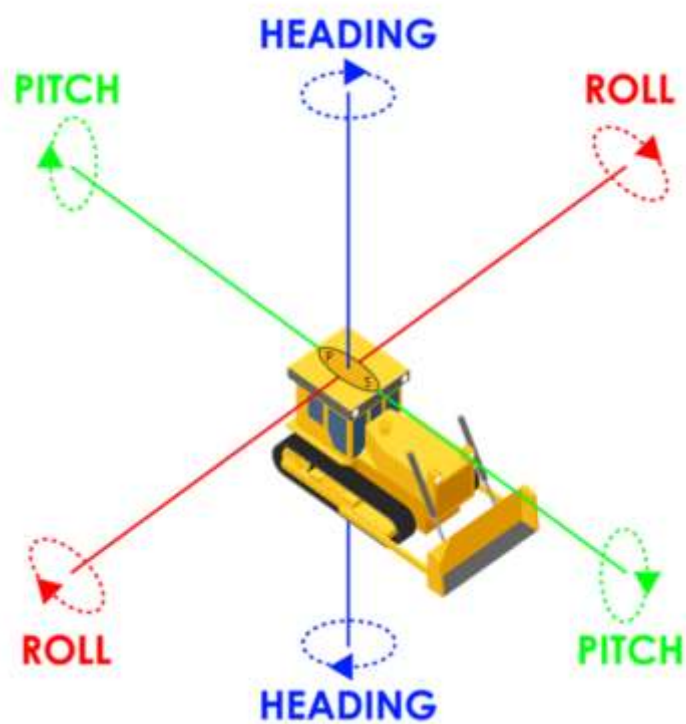
図 2-2 VR500 の設置方向と方位、ピッチ、ロールの値（中心軸方向に設置）
