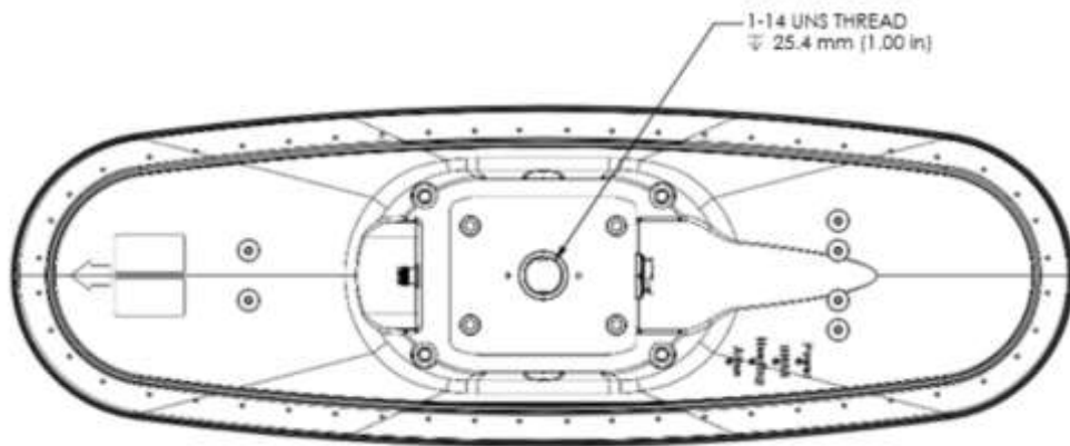
図 2-7 ポールマウントブラケット仕様
