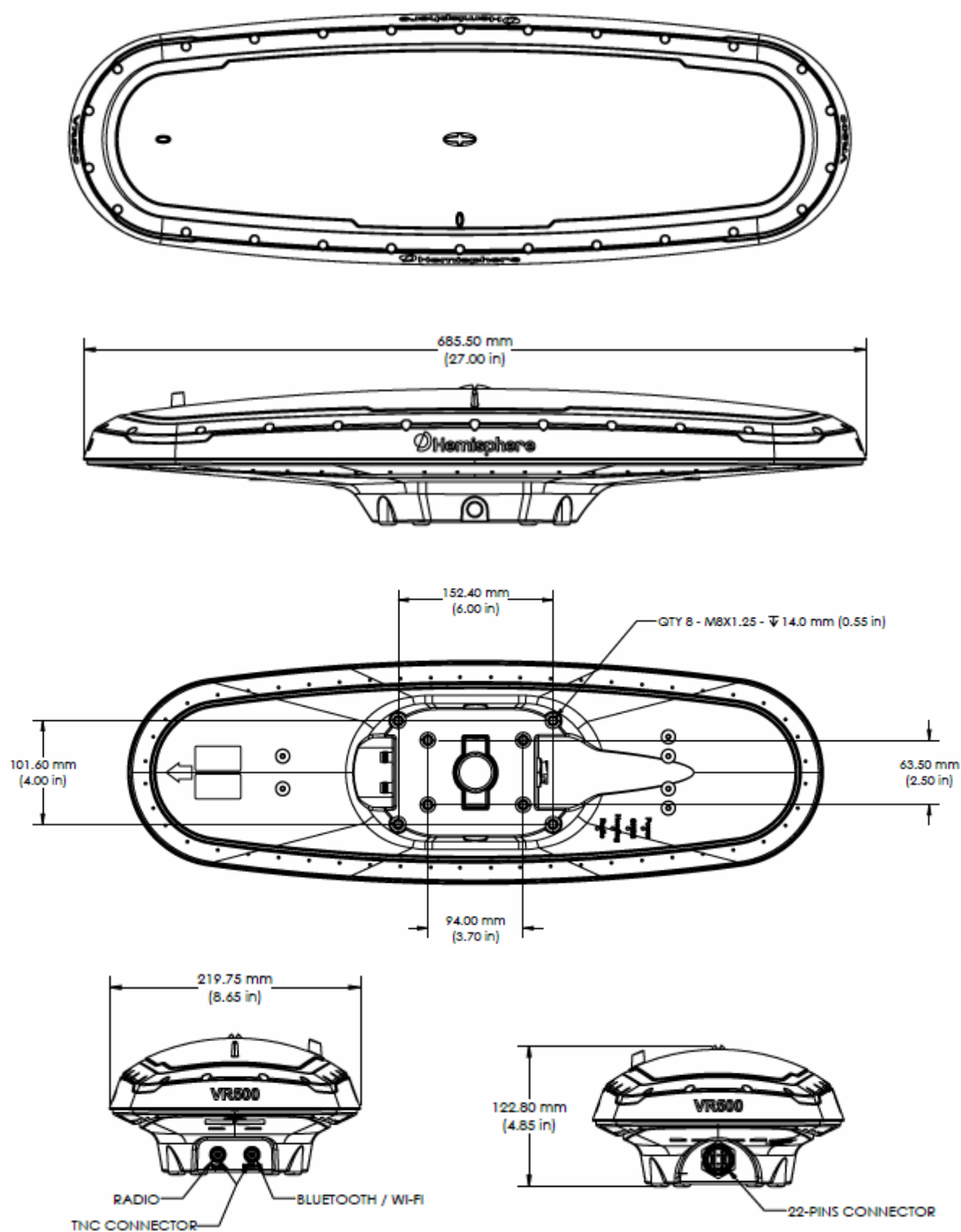
図 2-5 VR500 の寸法図
